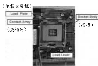
775 針插槽圖
